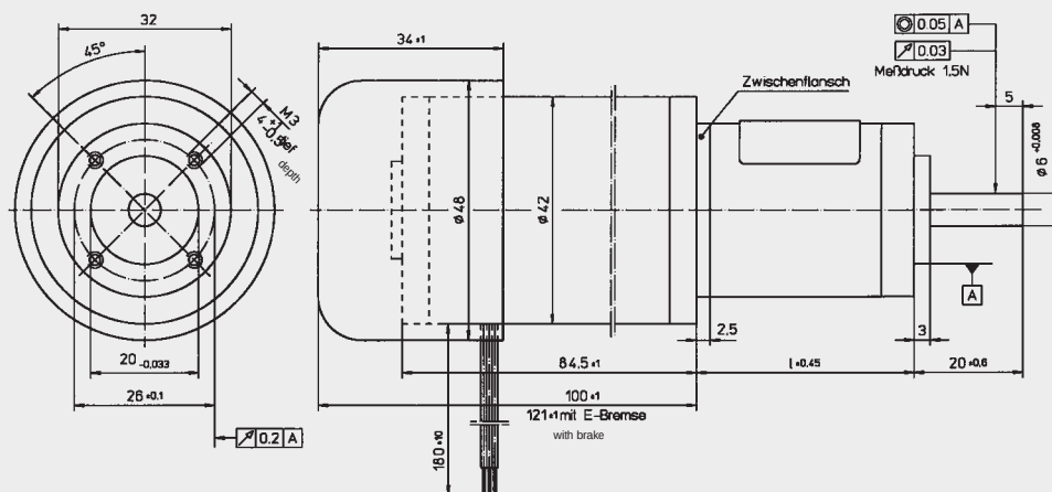
GEAR UNIT STAGES GETRIEBESTUFEN DIM. I MASS I 1stage 1stufig 31 2stage 2stufig 40 3stage 3stufig 50
